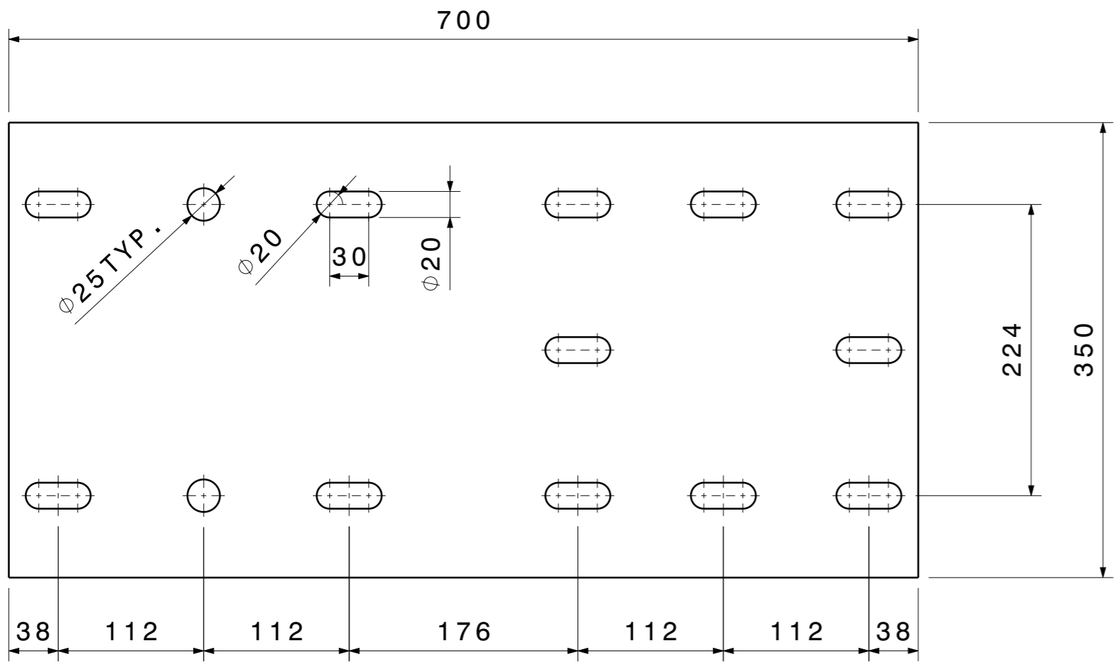
Top view Scale: 1:4
